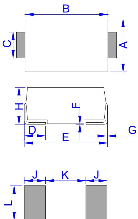
DO-214AB (SMC)
